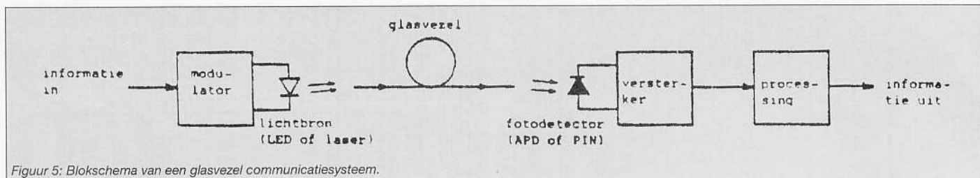
Figuur 5: Blokschema van een glasvezel communicatiesysteem.
