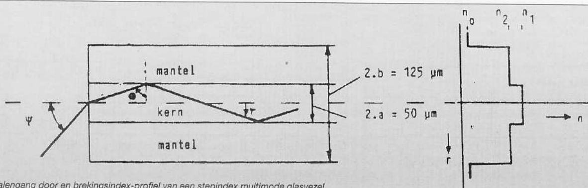
Figuur 4: Stralengang door en brekingsindex-profiel van een stepindex multimode glasvezel.
